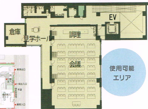
2階平面図
